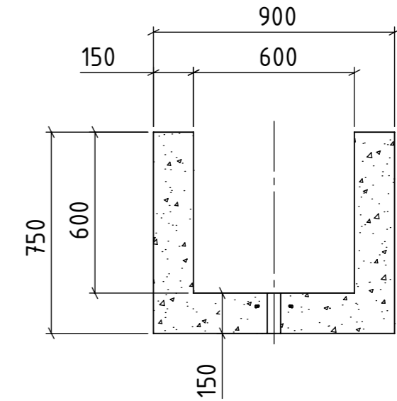
LEIKKAUS A-A
